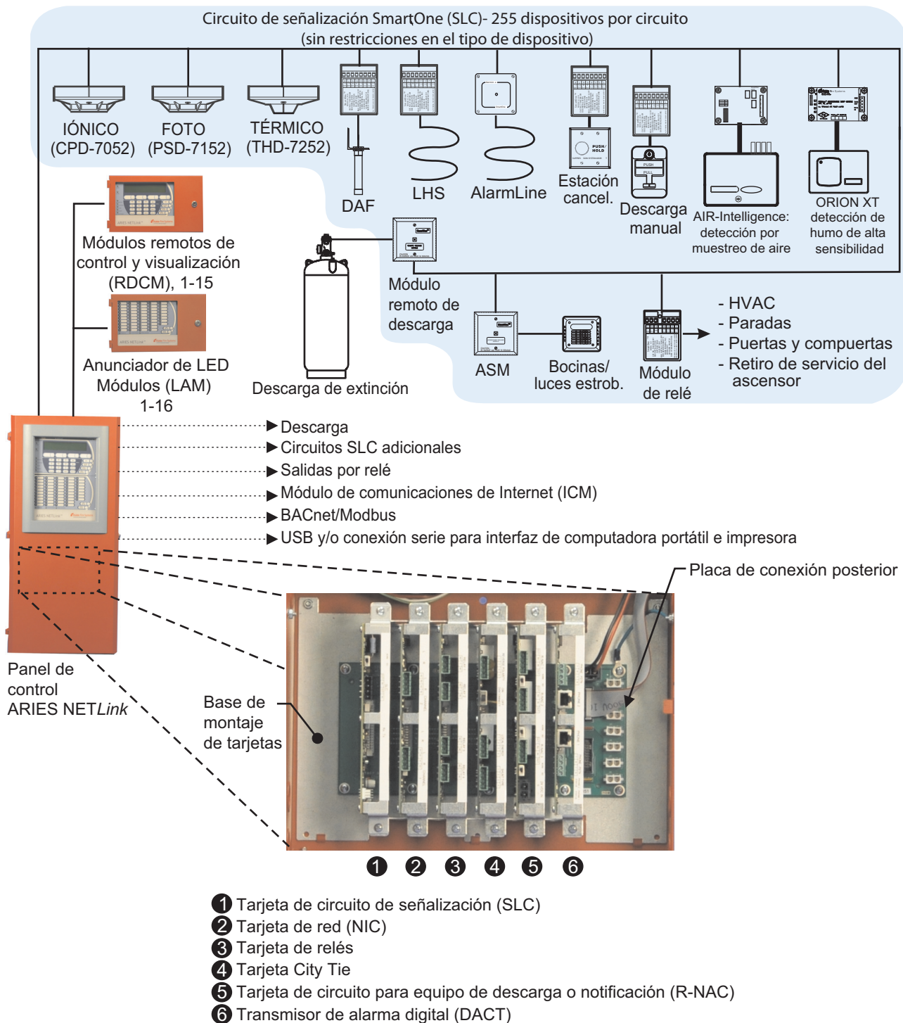
Figura 1. Diseño modular para cumplir con las aplicaciones más exigentes
